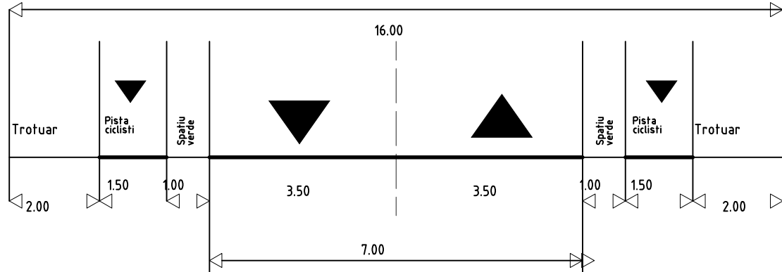
Profil propus - strada cat. III.6b - str. 1 Decembrie 1918
