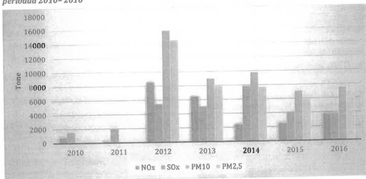
Figura 4-1: Tendința emisiilor totale de poluanți atmosferici, la nivelul județului Olt, pentru perioada 2010-2016
