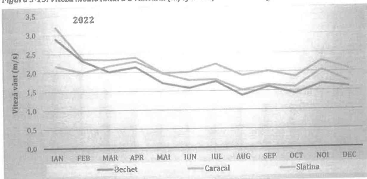
Figura 3-13: Viteza medie lunară a vântului (m/s) la stațiile meteorologice analizate, în anul 2022
