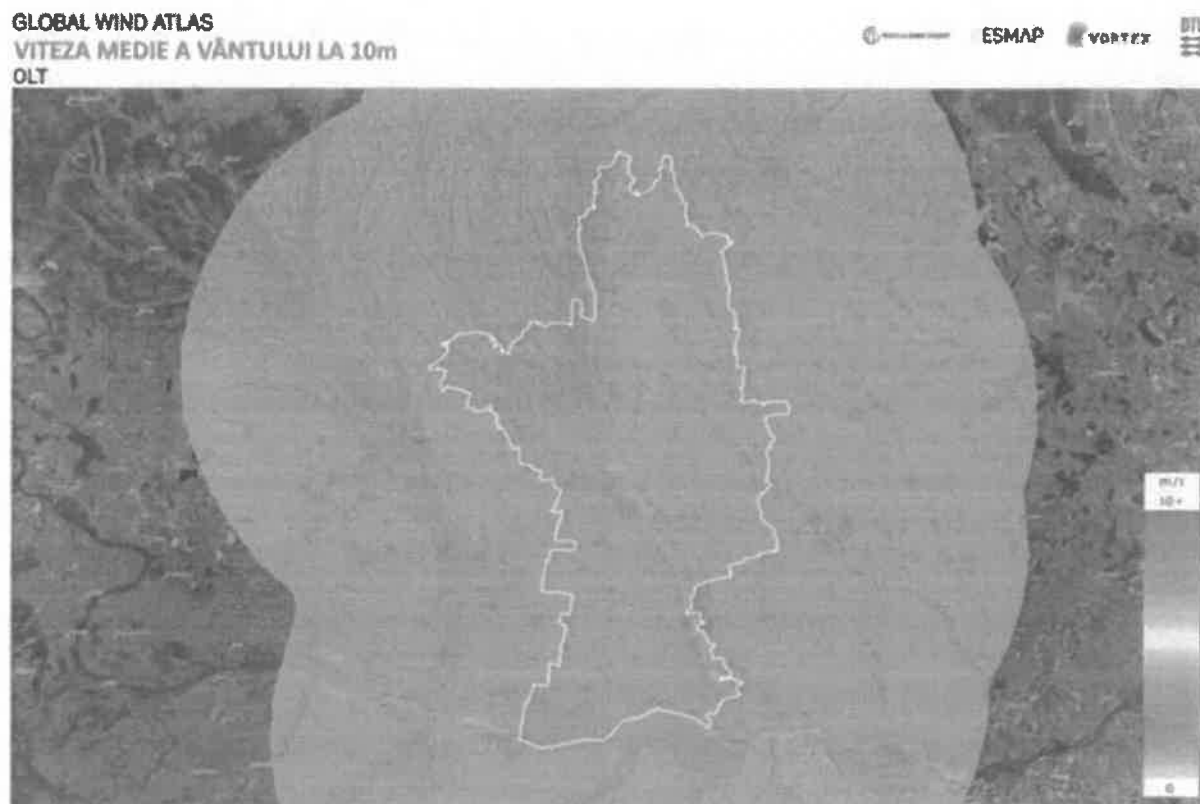
Figura 3-10: Harta vitezei medii a vântului la nivelul județului Olt
