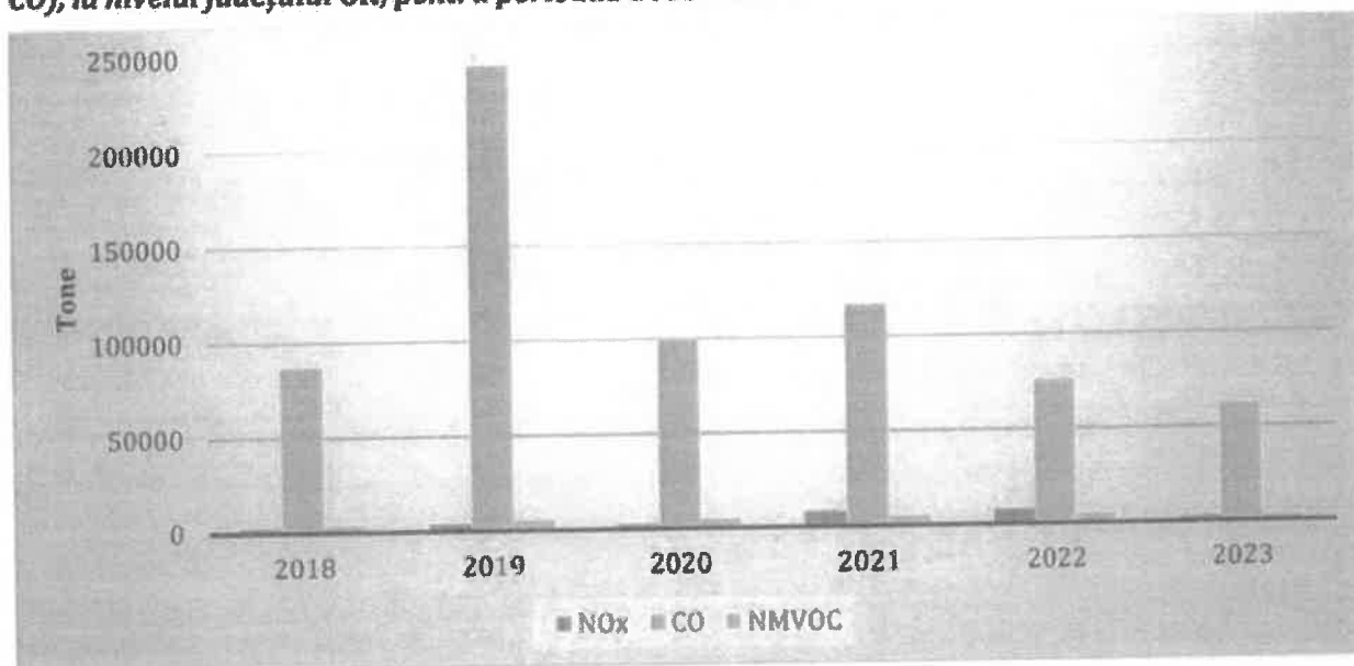
Figura 3-16: Tendința emisiilor totale de poluanți atmosferici precursori ai ozonului (NO x , NMVOC, CO), la nivelul județului Olt, pentru perioada 2018 - 2023
