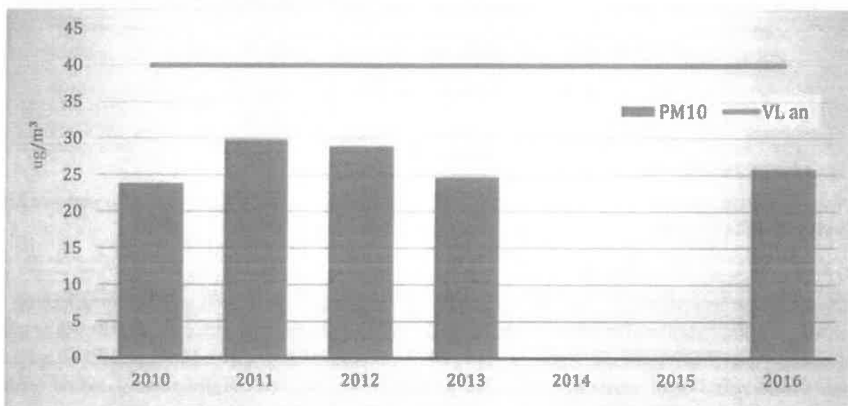
Figura 4-3: Evoluția concentrațiilor medii anuale pentru \text{PM}_{10} înregistrate la stația automată de monitorizare OT-1 în perioada 2010-2016
