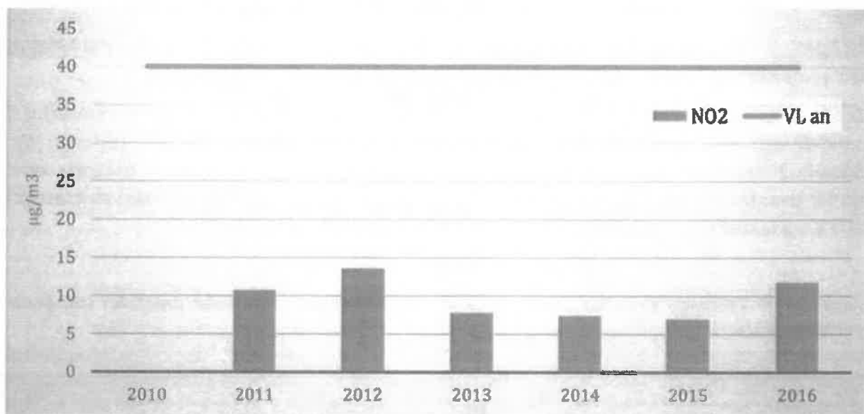
Figura 4-2: Evoluția concentrațiilor medii anuale pentru \text{NO}_2 înregistrate la stația automată de monitorizare OT-1 în perioada 2010 - 2016
