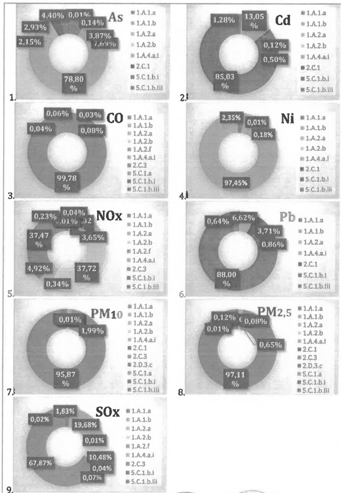
Figura 3-6: Contribuția sectoarelor de activitate (surse staționare) la emisiile totale de poluanți din județul Olt, în anul de referință 2022 (%)
