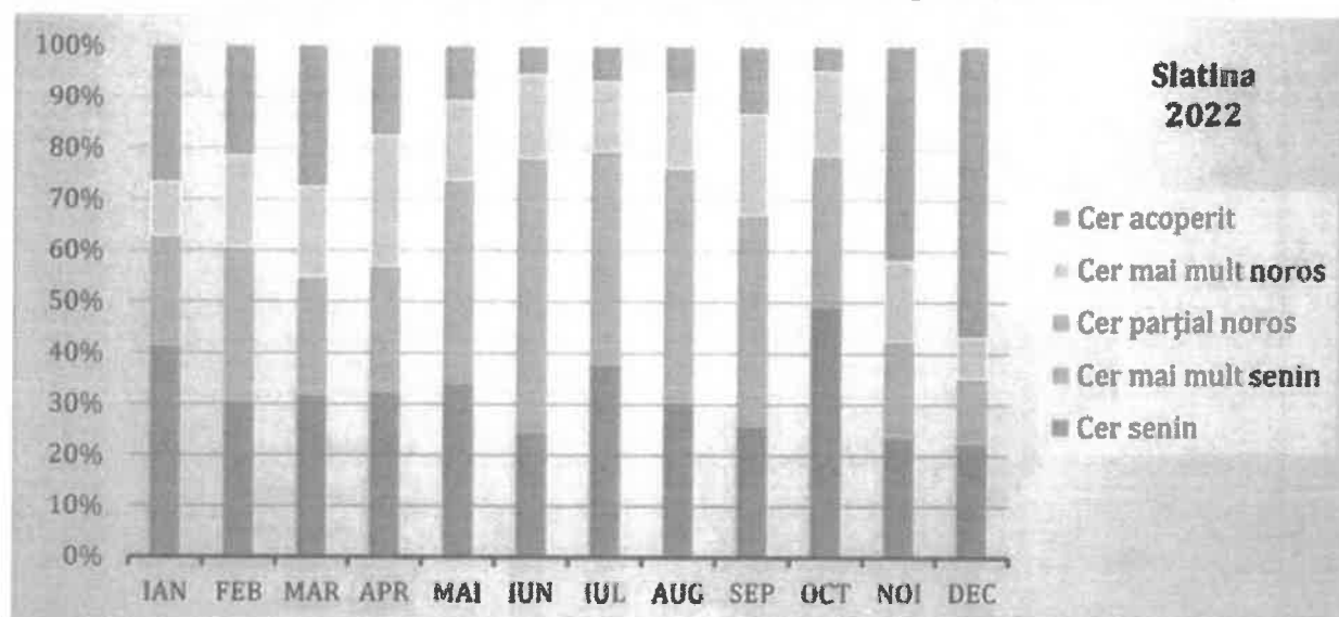
Figura 2-9: Nebulozitatea lunară înregistrată la stația meteorologică Slatina în anul 2022
