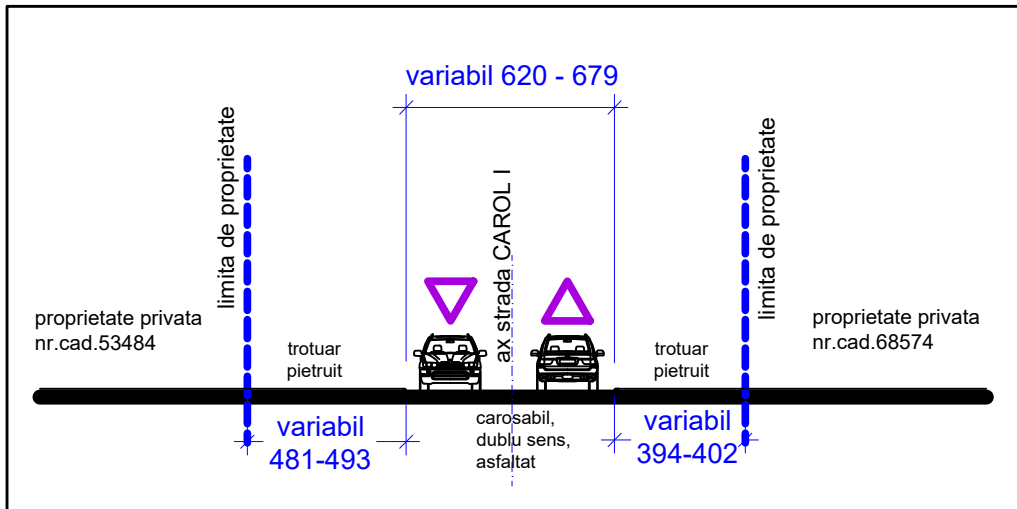
PROFIL 1-1 - CALE DE ACCES EXISTENTA (str.CAROL I)
